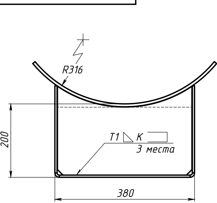
Поз.2 (Подушка)
