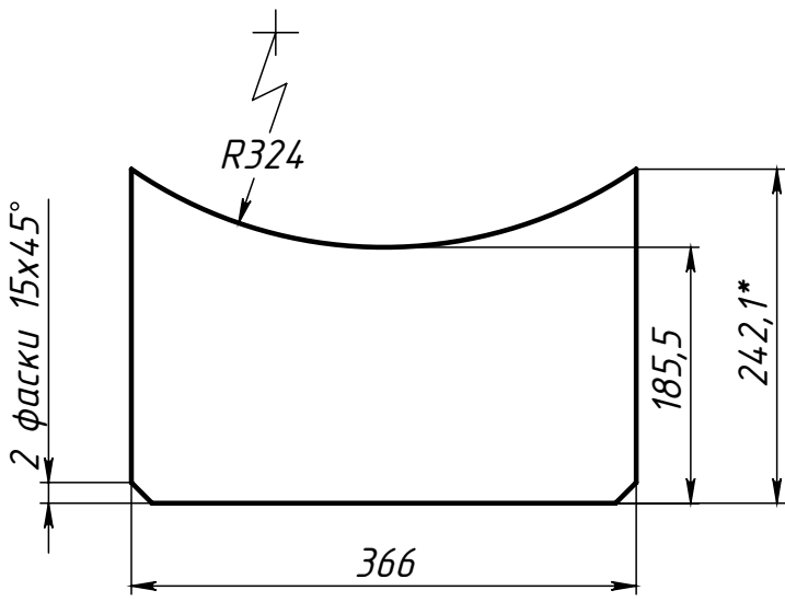
Поз.4 (Ребро)
