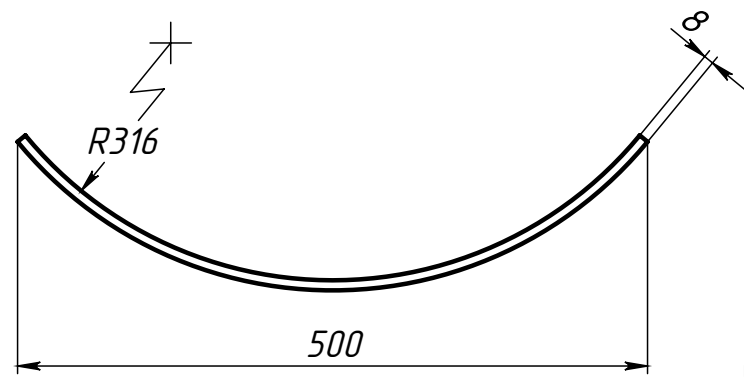
Поз.2 (Подушка)
